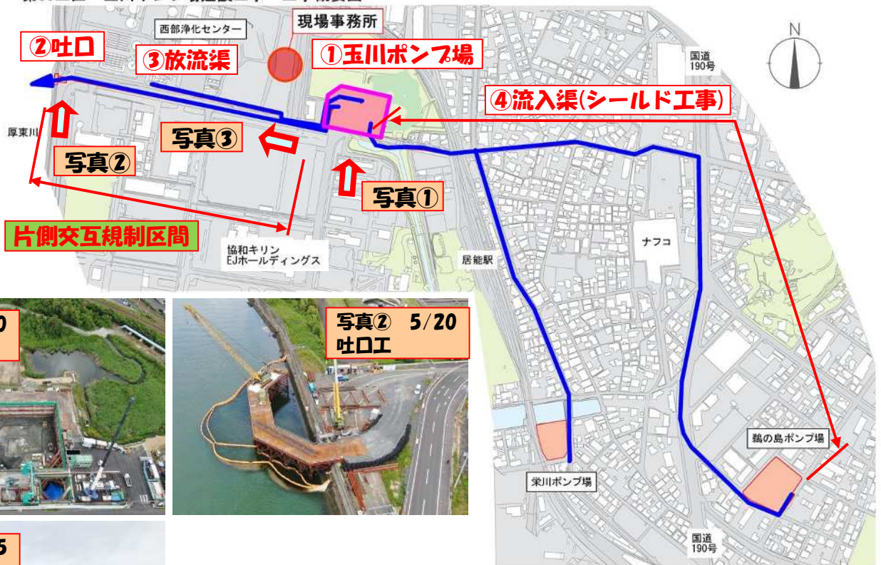
第80工区 玉川ポンプ場建設工事 工事概要図
